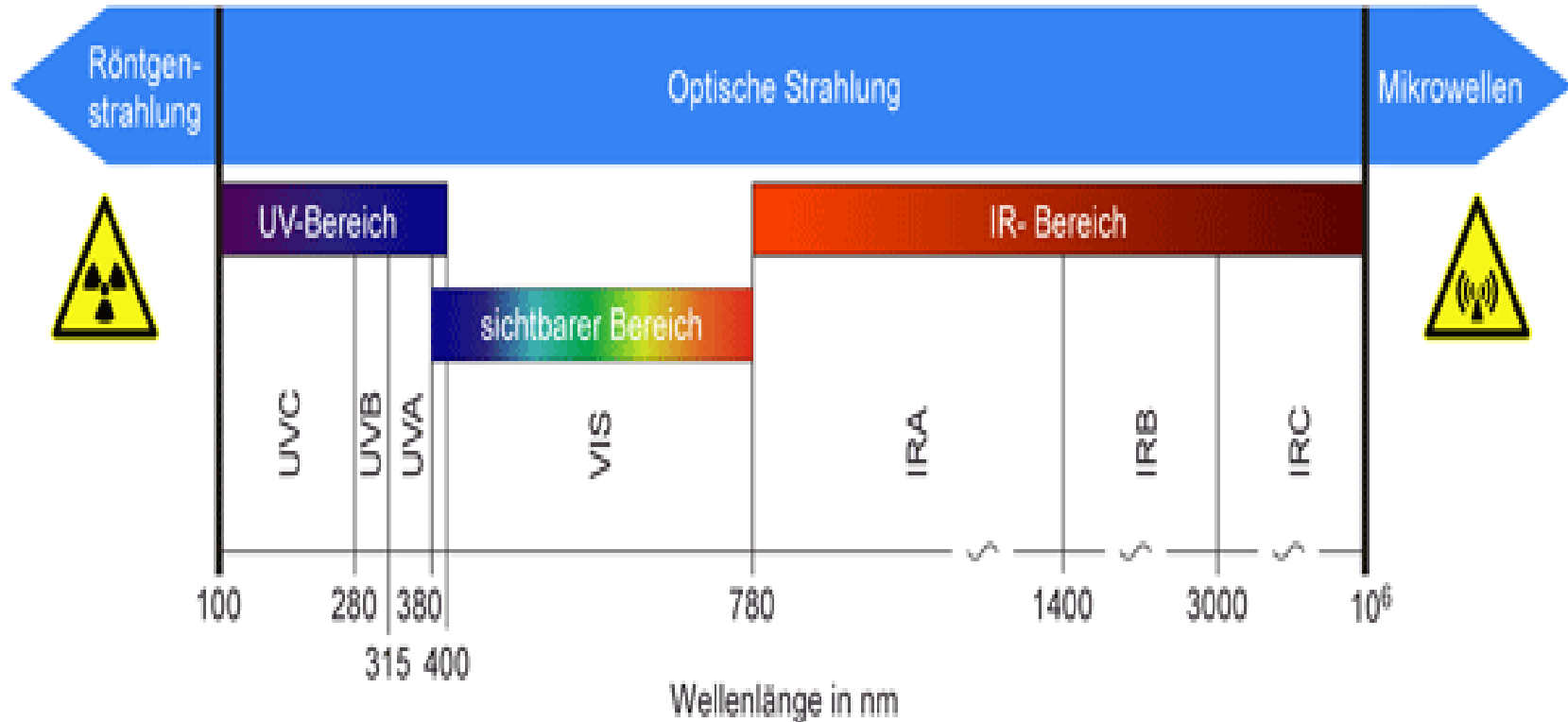
Elektromagnetisches Spektrum (Ausschnitt)
